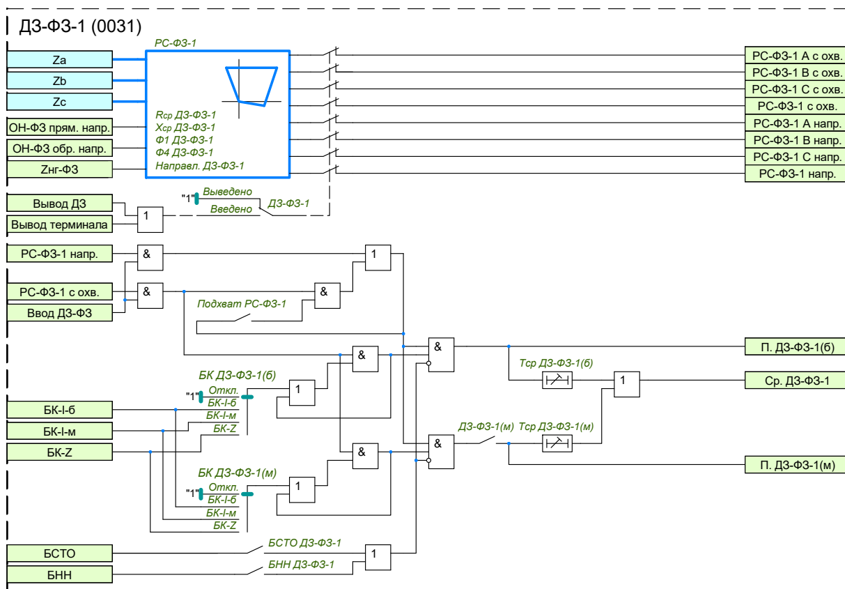
Рисунок 1.10 – Функциональная схема логики ДЗ-ФЗ-1
