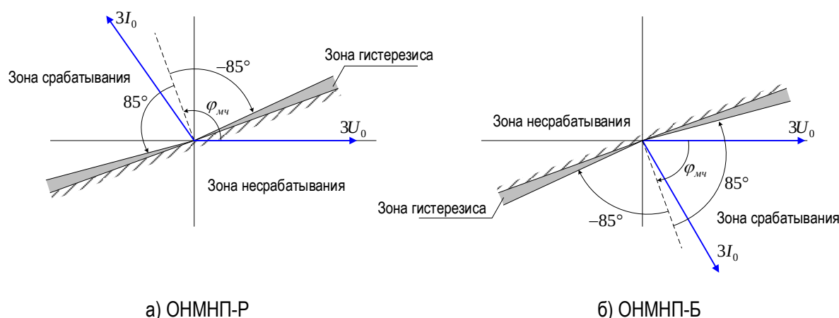
Рисунок 1.20 – Характеристики срабатывания ОНМП
