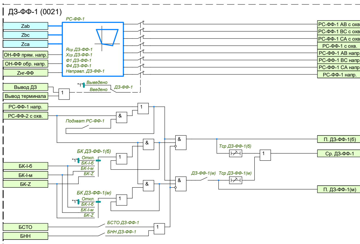
Рисунок 1.7 – Функциональная схема логики ДЗ-ФФ-1
