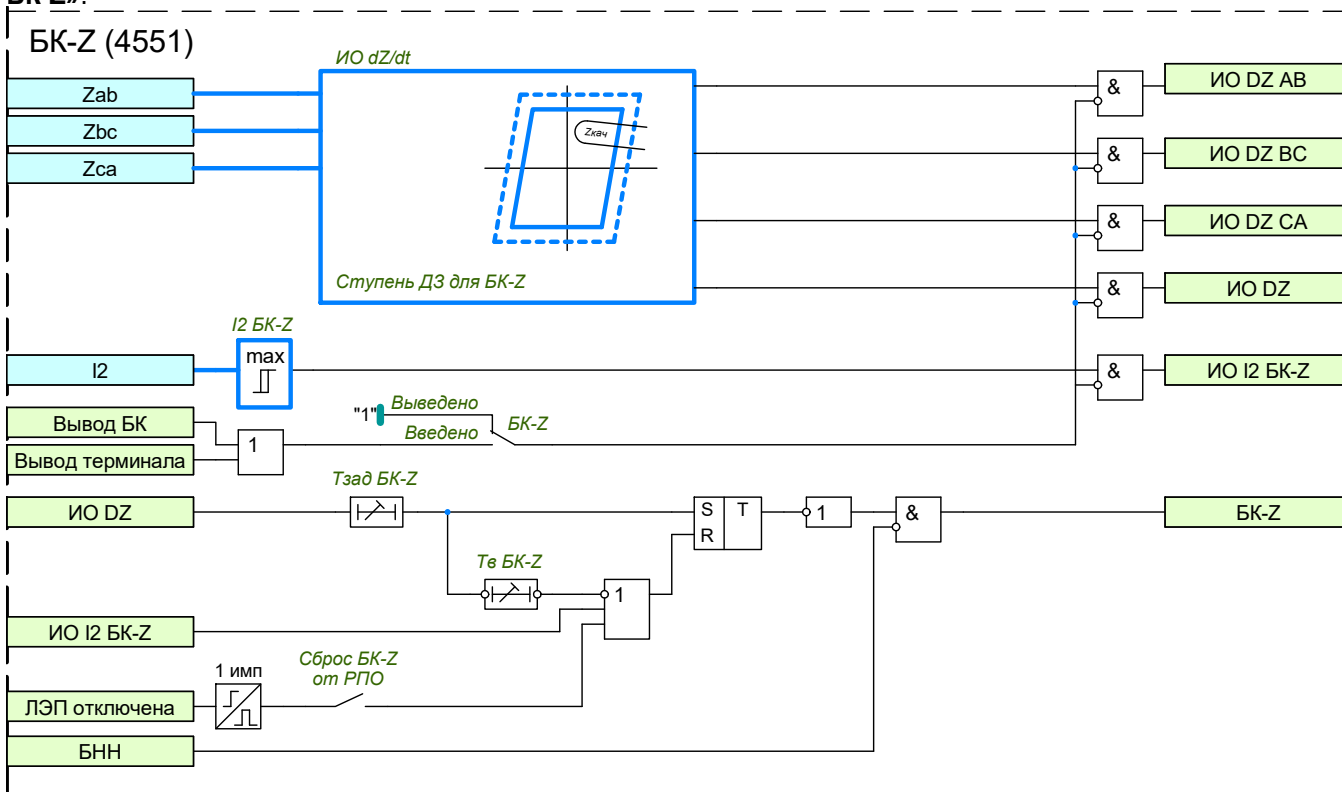
Рисунок 1.17 – Функциональная схема БК-Z
