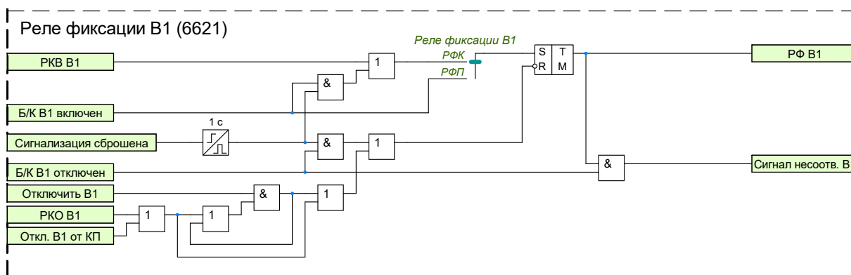
Рисунок 1.52 – Функциональная схема логики реле фиксации В1
