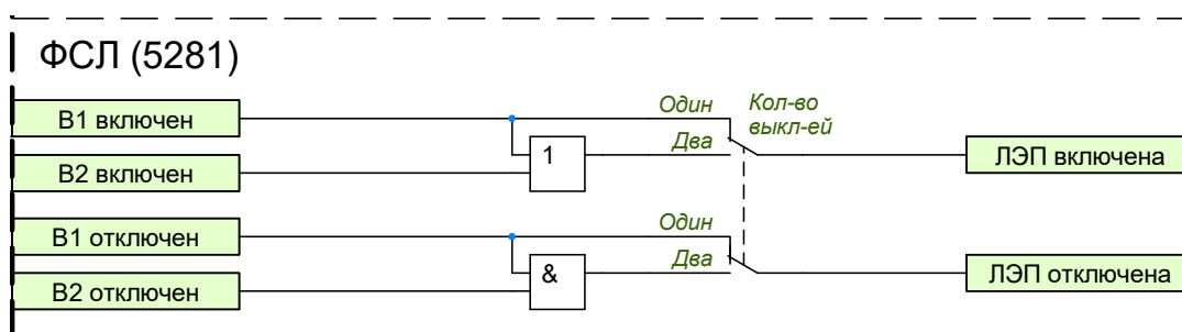
Рисунок 1.56 – Функциональная схема логики ФСЛ
