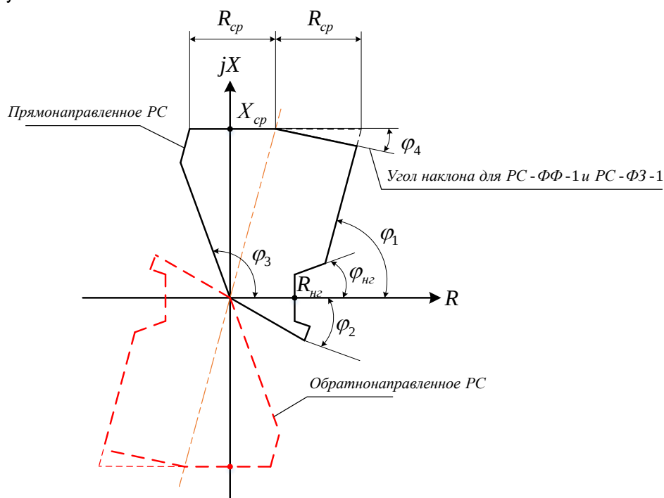
Рисунок 1.4 – Характеристики срабатывания направленного РС
