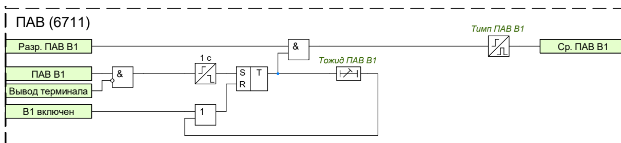
Рисунок 1.46 – Функциональная схема логики ПАВ В1
