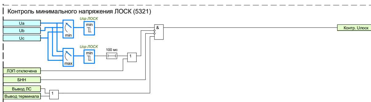
Рисунок 1.38 – Функциональная схема логики контроля минимального напряжения ЛОСК
