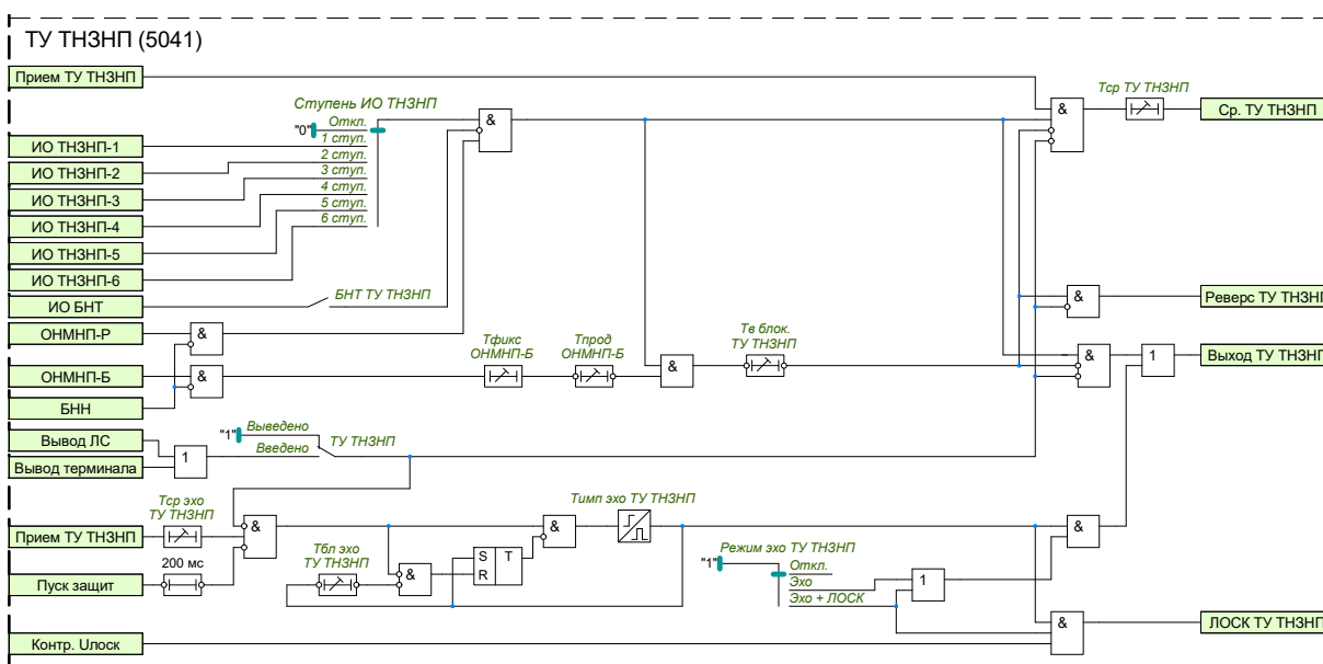
Рисунок 1.39 – Функциональная схема ТУ ТНЗНП
