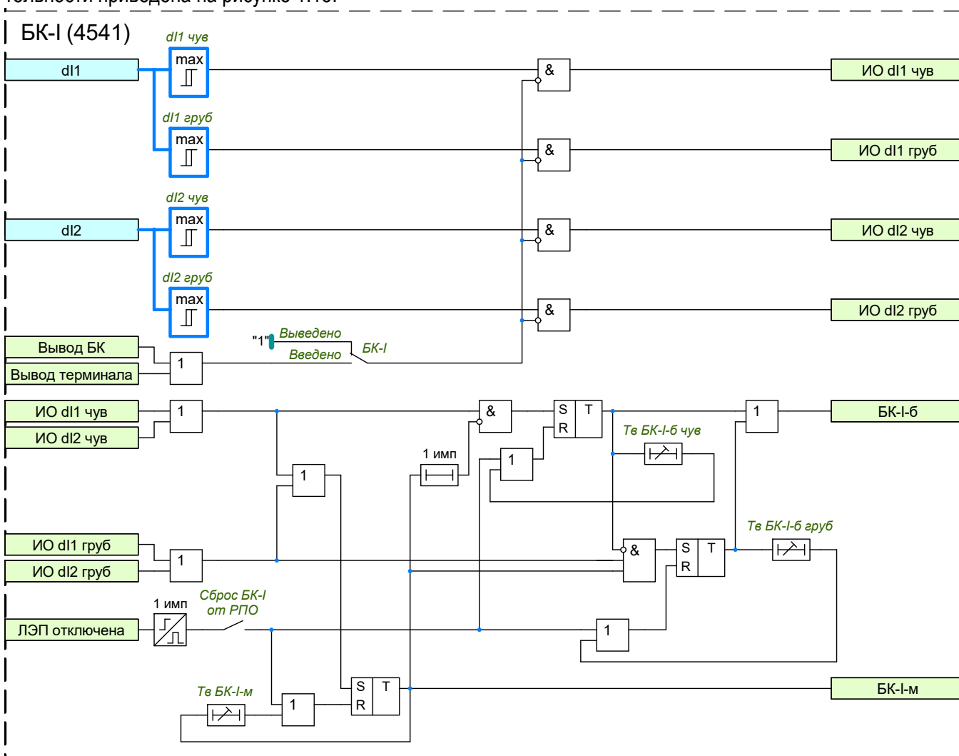
Рисунок 1.15 – Функциональная схема пуска БК-І
