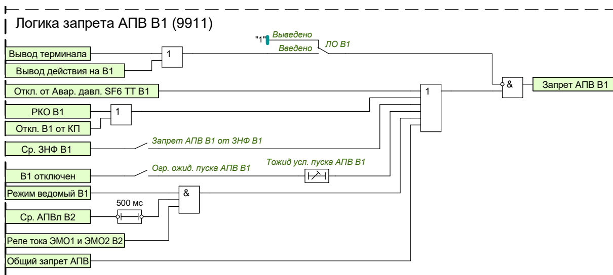
Рисунок 1.45 – Функциональная схема запрета АПВ В1
