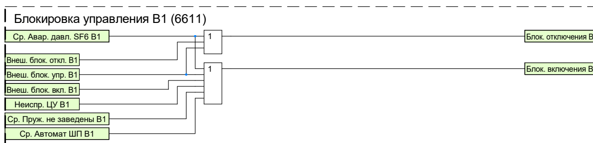
Рисунок 1.51 – Функциональная схема блокировки управления В1
