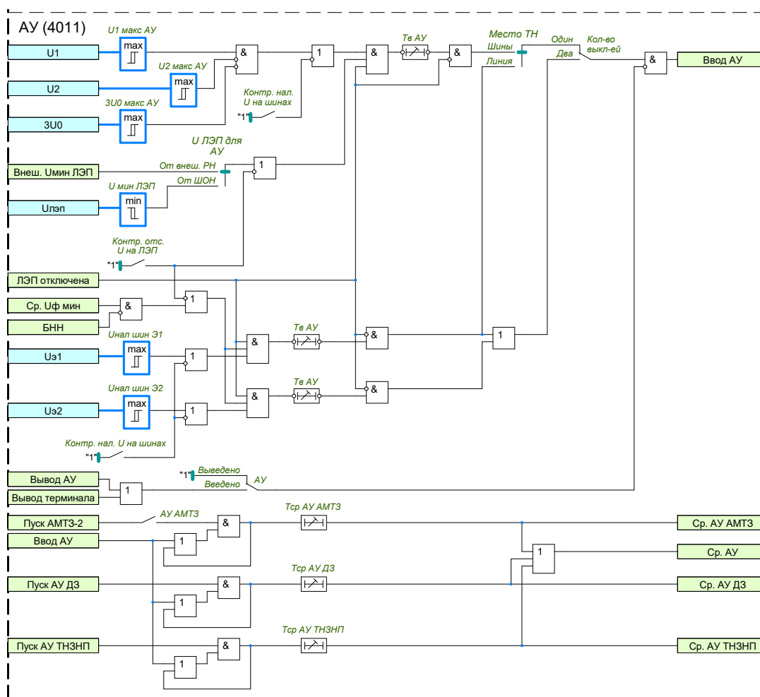
Рисунок 1.33 – Функциональная схема АУ
