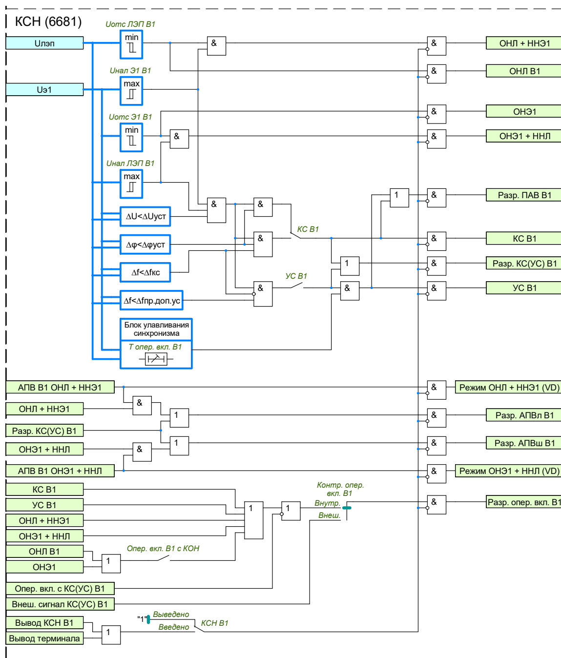
Рисунок 1.41 – Функциональная схема логики КСН В1
