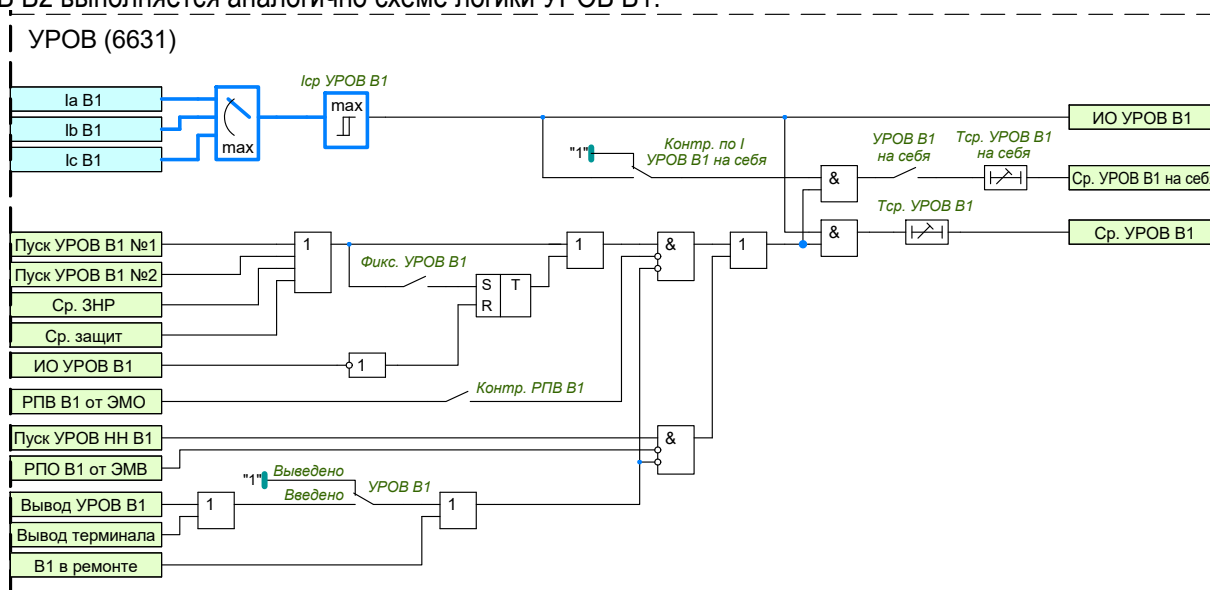
Рисунок 1.40 – Функциональная схема логики УРОВ В1
