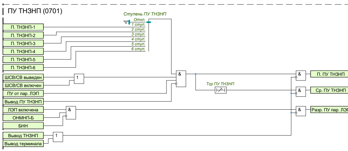
Рисунок 1.24 – Функциональная схема пуска ПУ ТНЗНП
