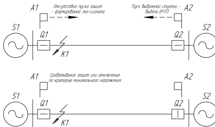
Рисунок 1.37 – Пояснение к принципу действия эхо-логики
