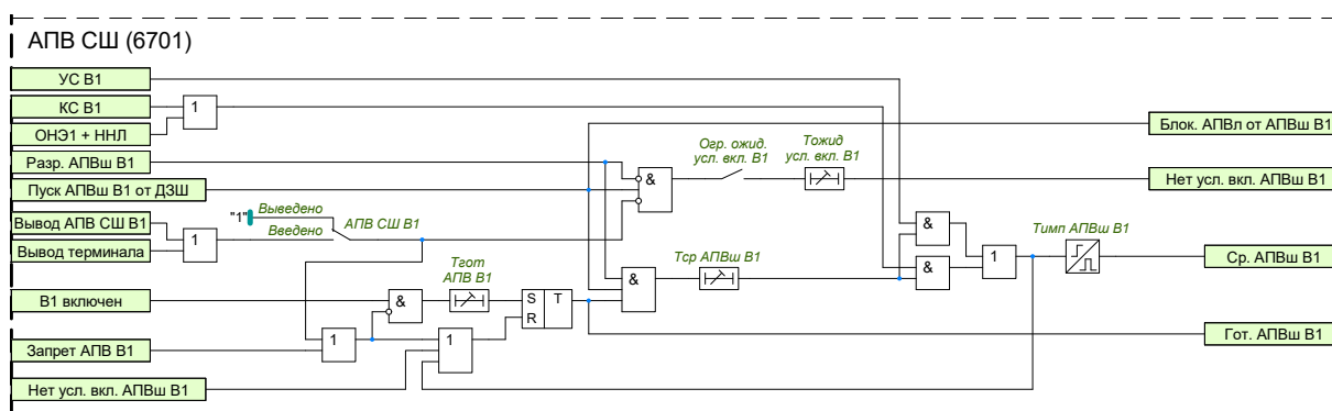
Рисунок 1.43 – Функциональная схема АПВ В1 СШ
