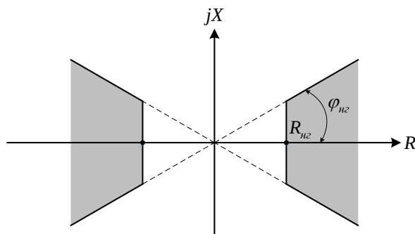
Рисунок 1.3 – Характеристика срабатывания измерительного органа отстройки от нагрузки
