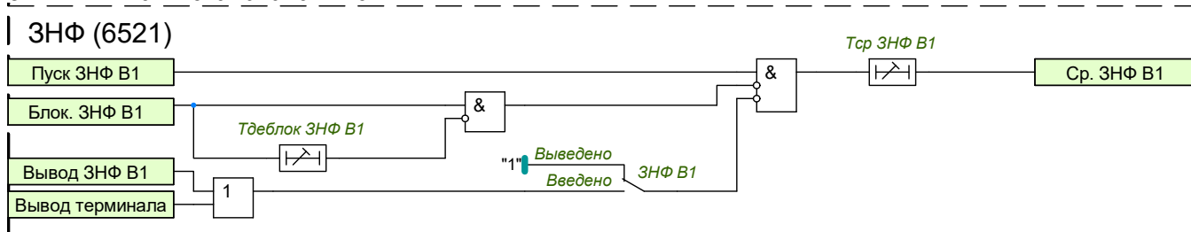
Рисунок 1.30 – Функциональная схема ЗНФ В1
