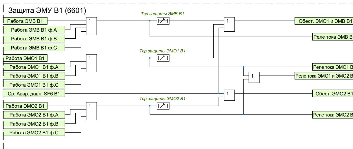
Рисунок 1.50 – Функциональная схема защиты ЭМУ В1
