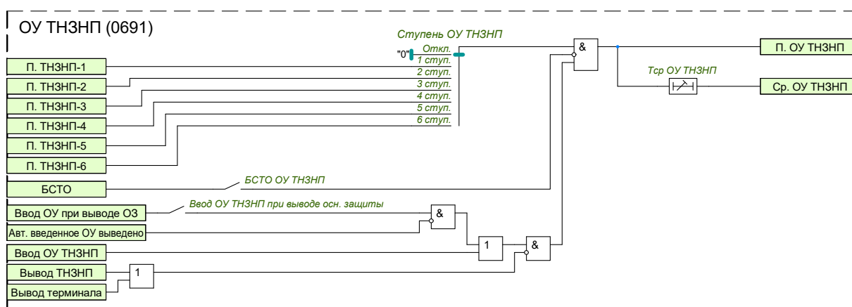
Рисунок 1.22 – Функциональная схема ОУ ТНЗНП
