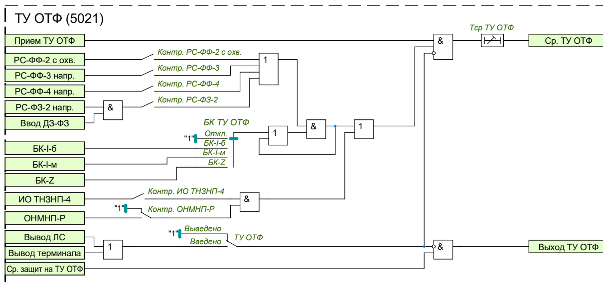
Рисунок 1.35 – Функциональная схема логики ТУ ОТФ
