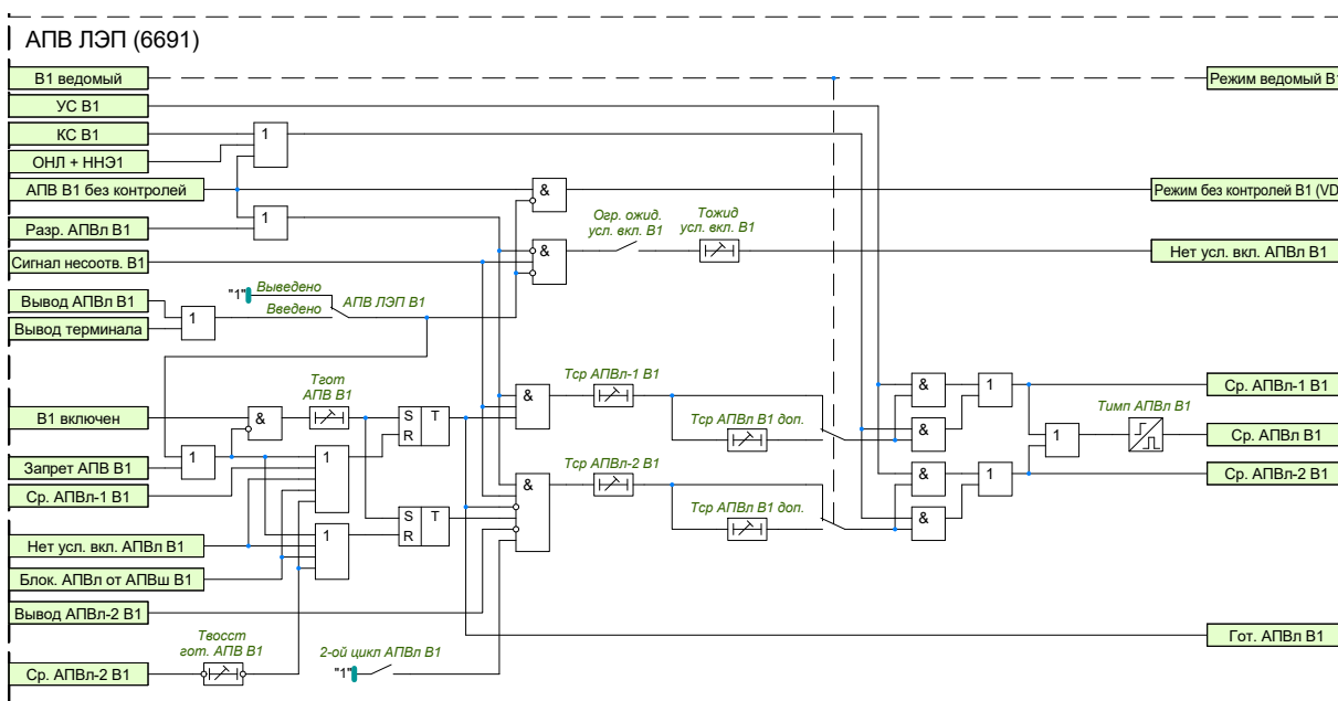
Рисунок 1.42 – Функциональная схема логики АПВ В1 ЛЭП
