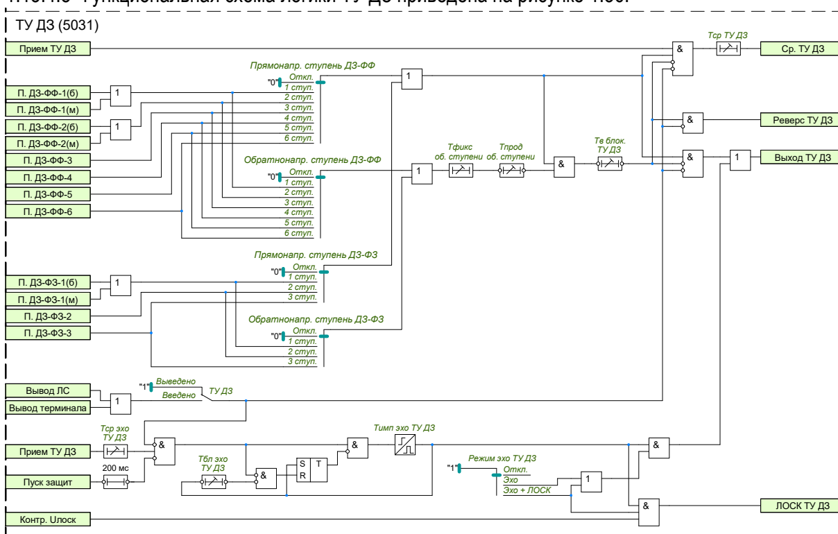
Рисунок 1.36 – Функциональная схема логики ТУ ДЗ
