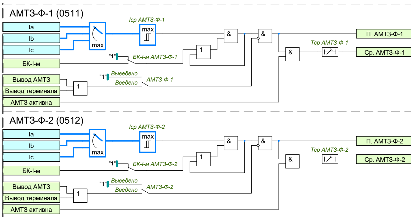
Рисунок 1.26 – Функциональная схема ступеней АМТЗ-Φ-1(2)
