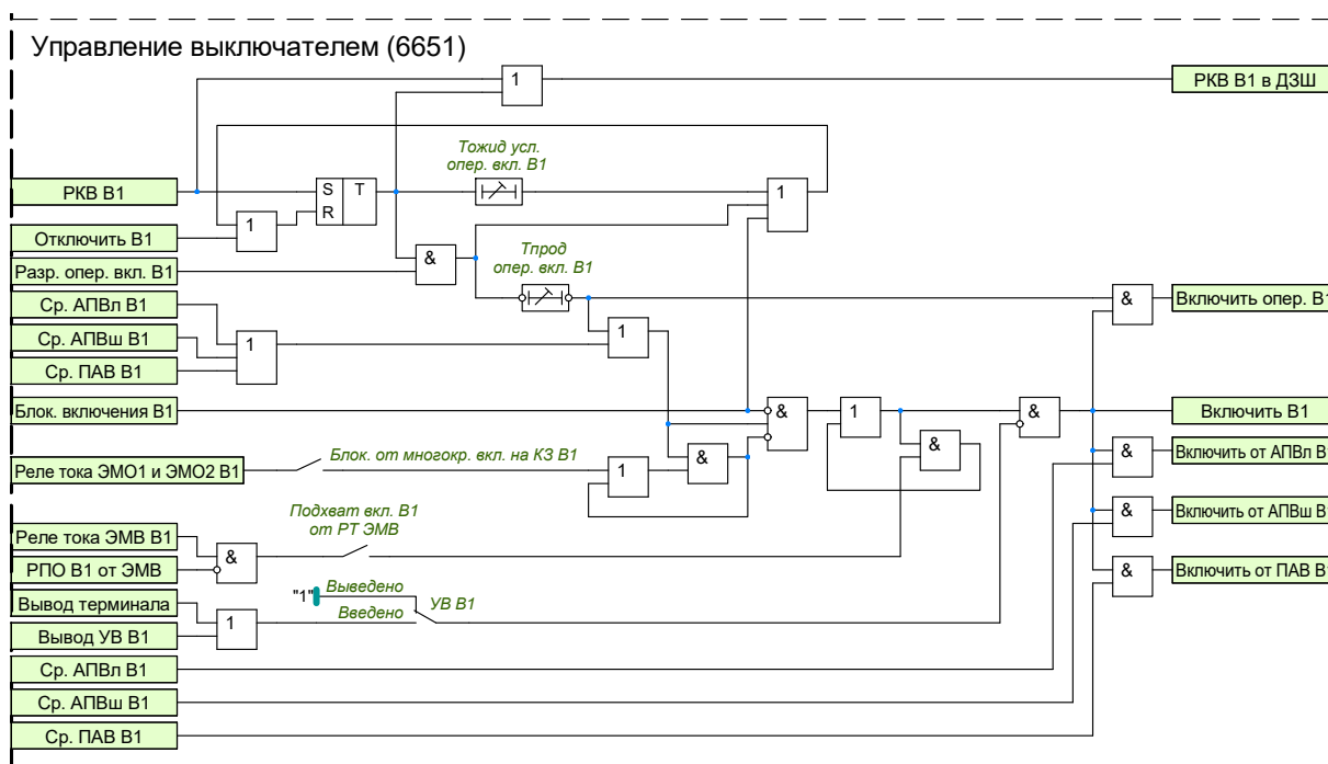
Рисунок 1.54 – Функциональная схема управления выключателем В1
