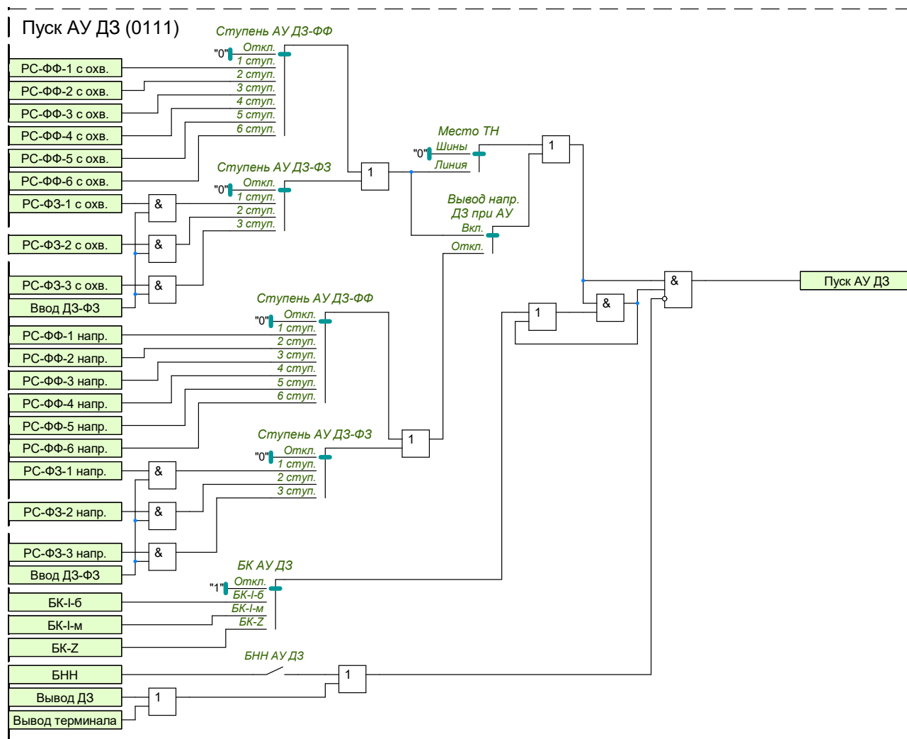
Рисунок 1.12 – Функциональная схема пуска АУ ДЗ
