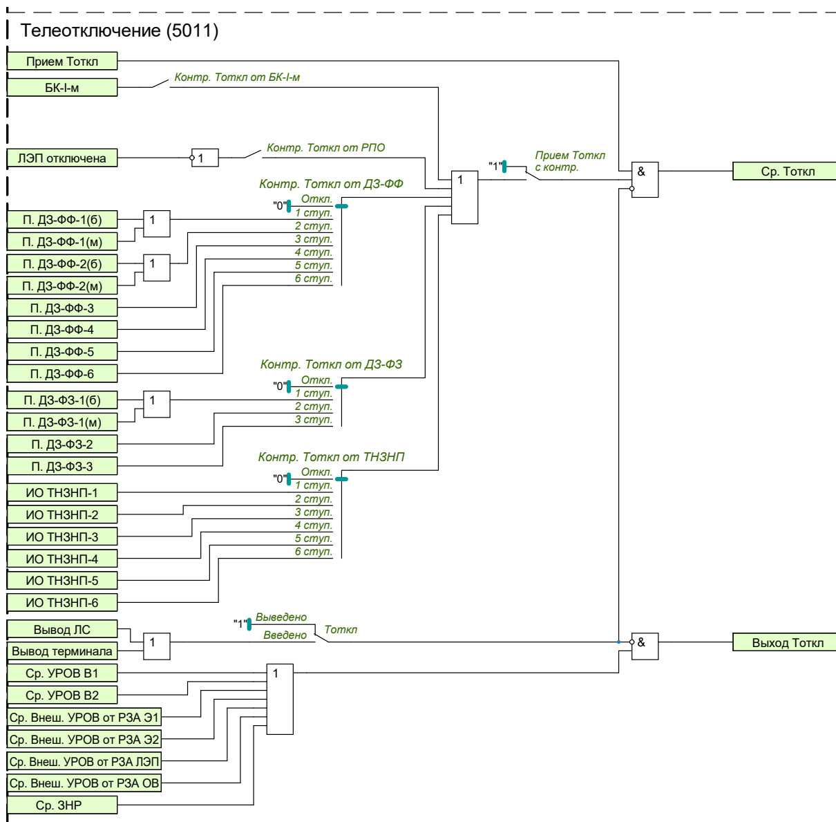
Рисунок 1.34 – Функциональная схема логики телеотключения
