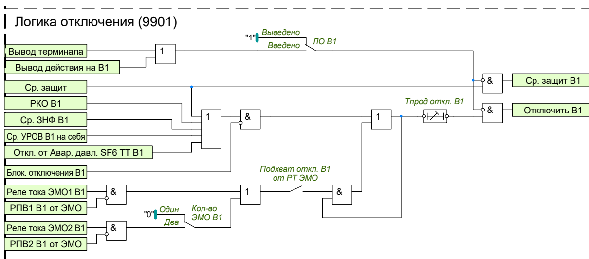
Рисунок 1.53 – Функциональная схема логики отключения В1
